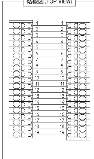
結線図 (TOP VIEW)
