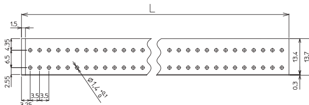
基板取り付け穴寸法図 (TOP VIEW)
